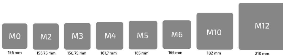
〈태양전지용 웨이퍼 크기 비교〉
